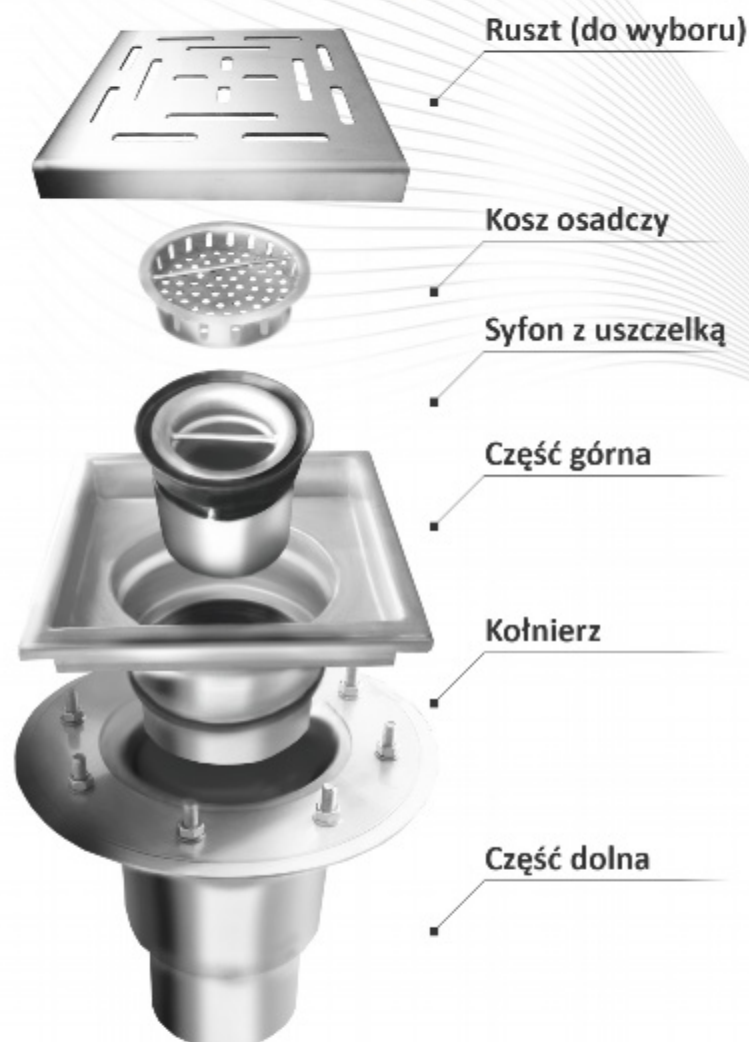
WPUST SEMI-PROF KMB STEEL PRODUCT (2 moduły)
